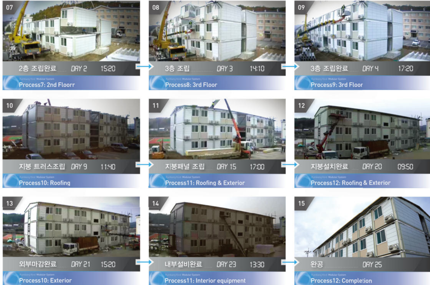
독신숙소 모듈러 시공현장
